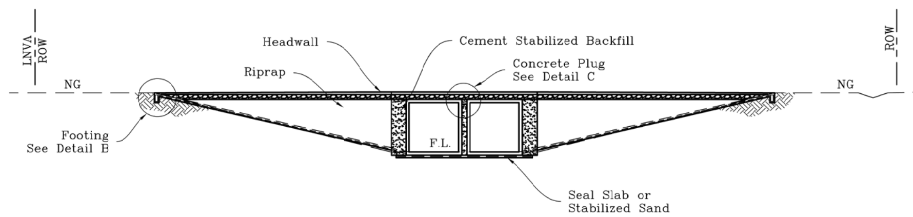
Rock Drive - (2) 10'X10'X80' Concrete Box Culverts STA 76+98
